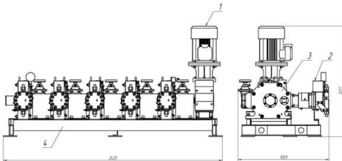
Рис. 1 - Строение блочного агрегата серии AP45
